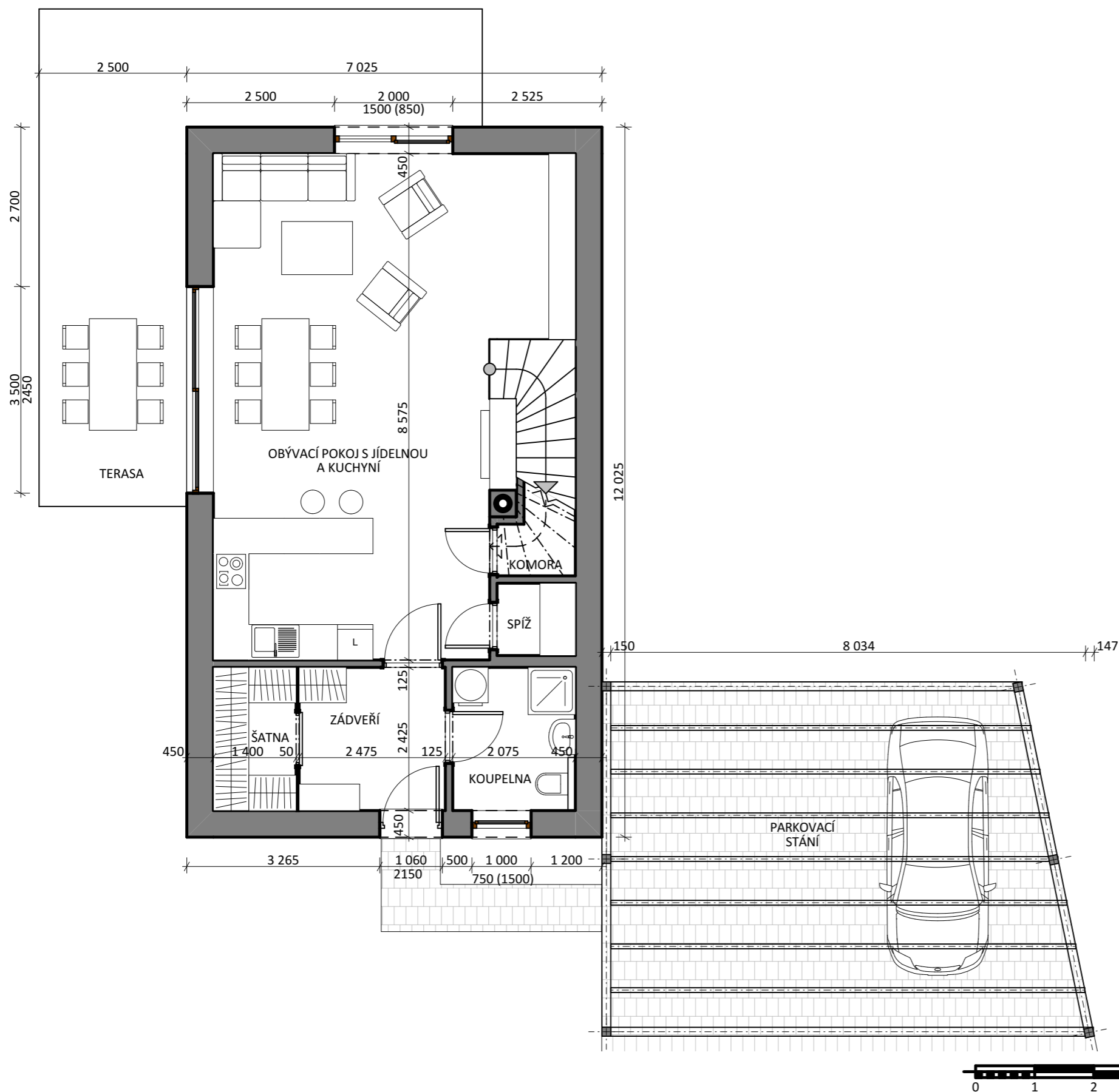
Půdorys přízemí
